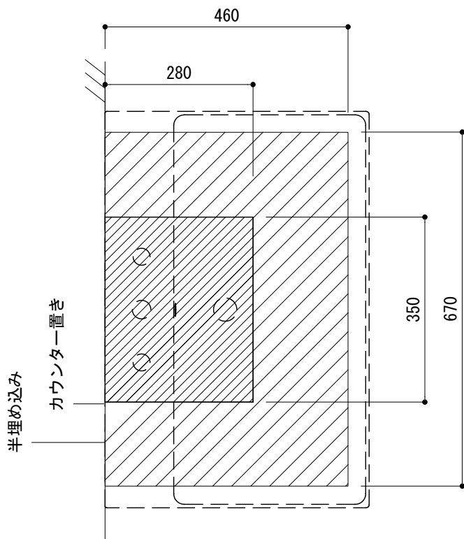
カウンター切込寸法
