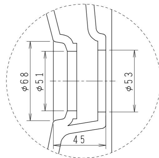
詳細図
