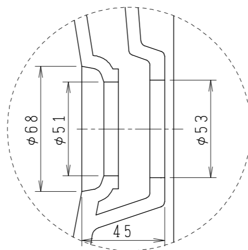
詳細図
