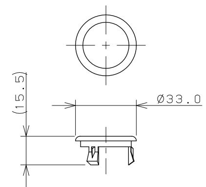
オーバーフローキャップ (×1)
